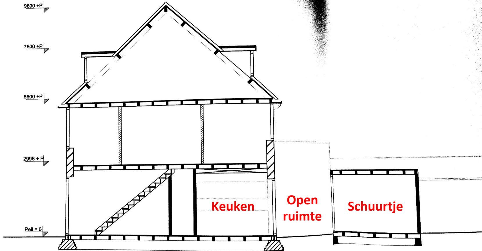
Doorsnede A - A
